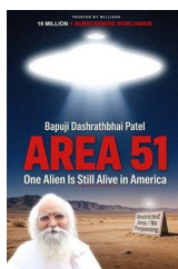
Area 51
