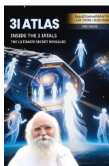
3i Atlas
